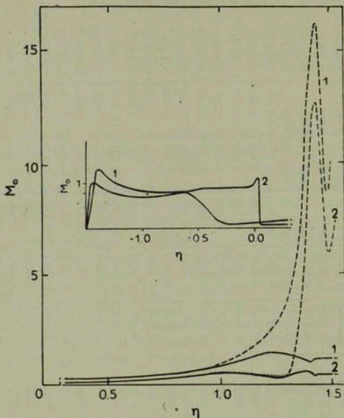
Рис. 1. Зависимость массы конфигураций из вырожденной плазмы от центрального давления ( \eta = \arctg \lg P_c / 10^{33} ) с учетом (кривая 2) и без учета пионизации (кривая 1).
