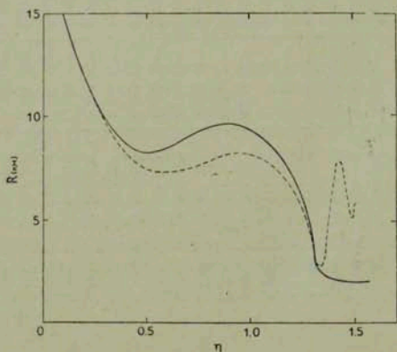
Рис. 2. Зависимость координатного радиуса от центрального давления ( \eta = \arctg \lg P_c / 10^{33} ). Пунктирная кривая относится к биметрической теории.
