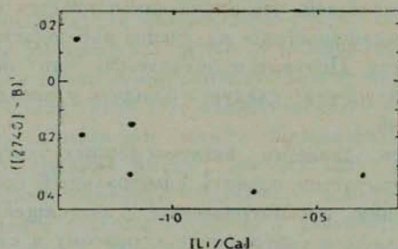
Рис. 2. По оси абсцисс — то же, что и на рис. 1, по оси ординат — исправленные межзвездное поглощение цвета ([2740] - B)' .
