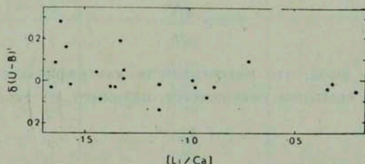
Рис. 1. По оси абсцисс отложены [Li/Ca] — логарифмы отношения содержания атомов лития к содержанию атомов кальция минус логарифм того же отношения для Солнца. По оси ординат — избытки цвета \delta(U-B)' .
